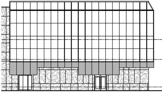
EXISTING WEST ELEVATION S. MAIN ST. SCALE: 1/8" = 1'-0"
